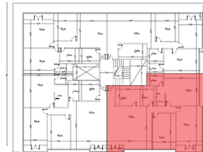
معماري الدور الثاني - الثالث - الرابع
