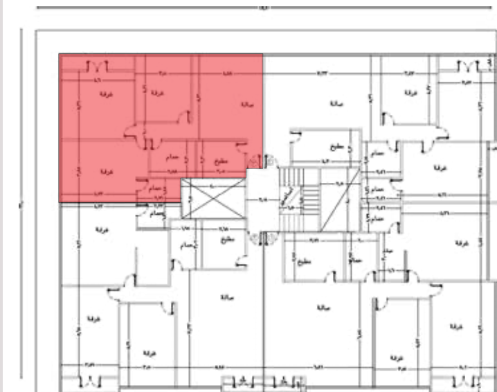
معماري الاول علوي
